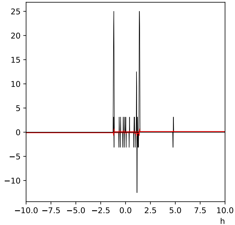
\chi_L(H) réseau de taille L=4 à T=1.5
