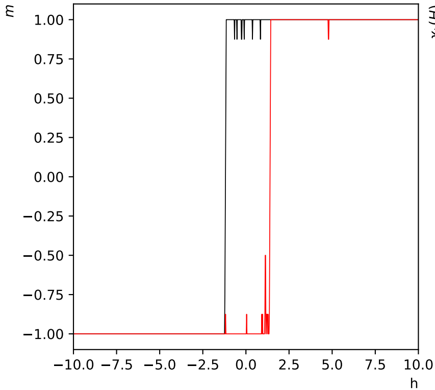
Hystérésis de l'aimantation réseau de taille L=4 - h=10 à T=1.5
